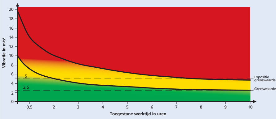
Grenswaarden voor vibratiebelastingen
