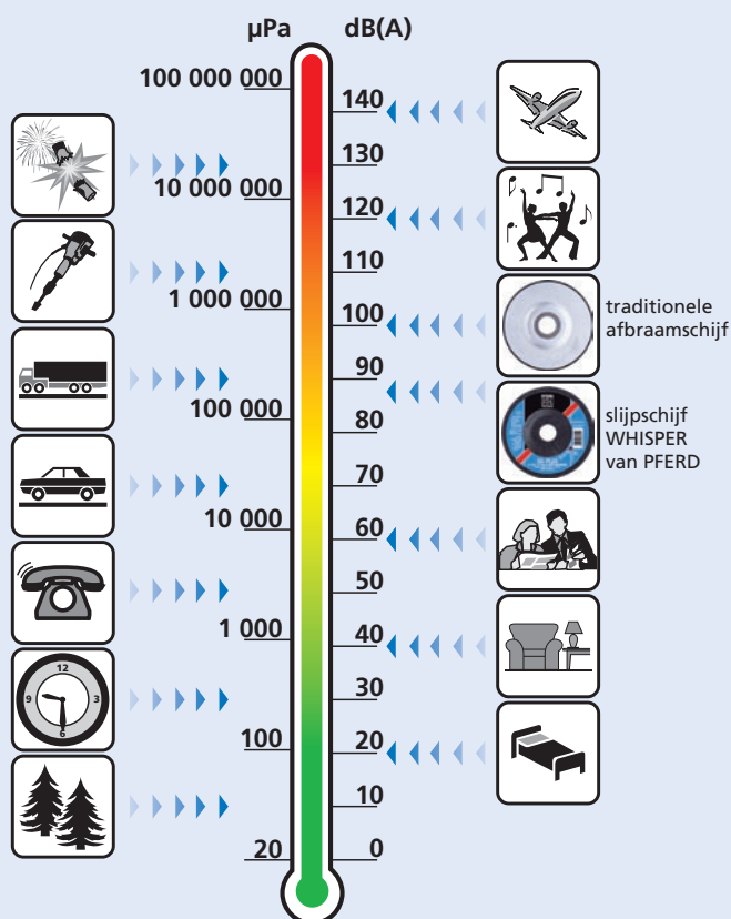
Voorbeelden van lawaai - geluidsdrumniveau
