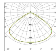
H00210 (120°)
