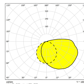
GALGO-LED in asymmetrische optiek.
