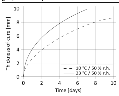
Schema 1: Uithardingsnelheid voor Sikaflex®-296
