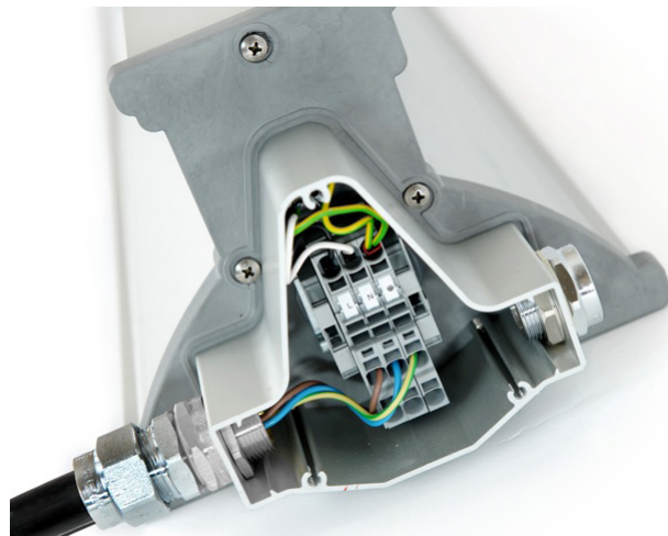
Klemmenstrook in de aansluitbox
